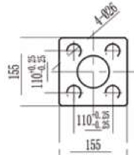
标准方法兰 Standard Square Flange
