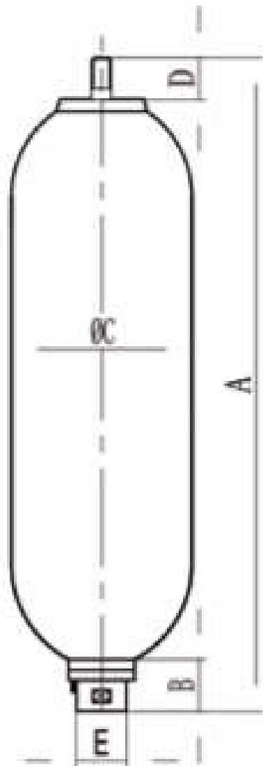
S-标准型 Standard Type
