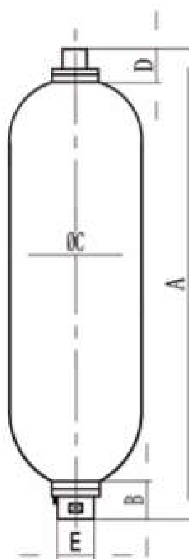
TR-顶部可修型 Top Repairable Type
