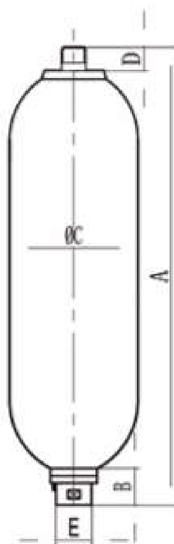
SB-标准型 Standard B Type
